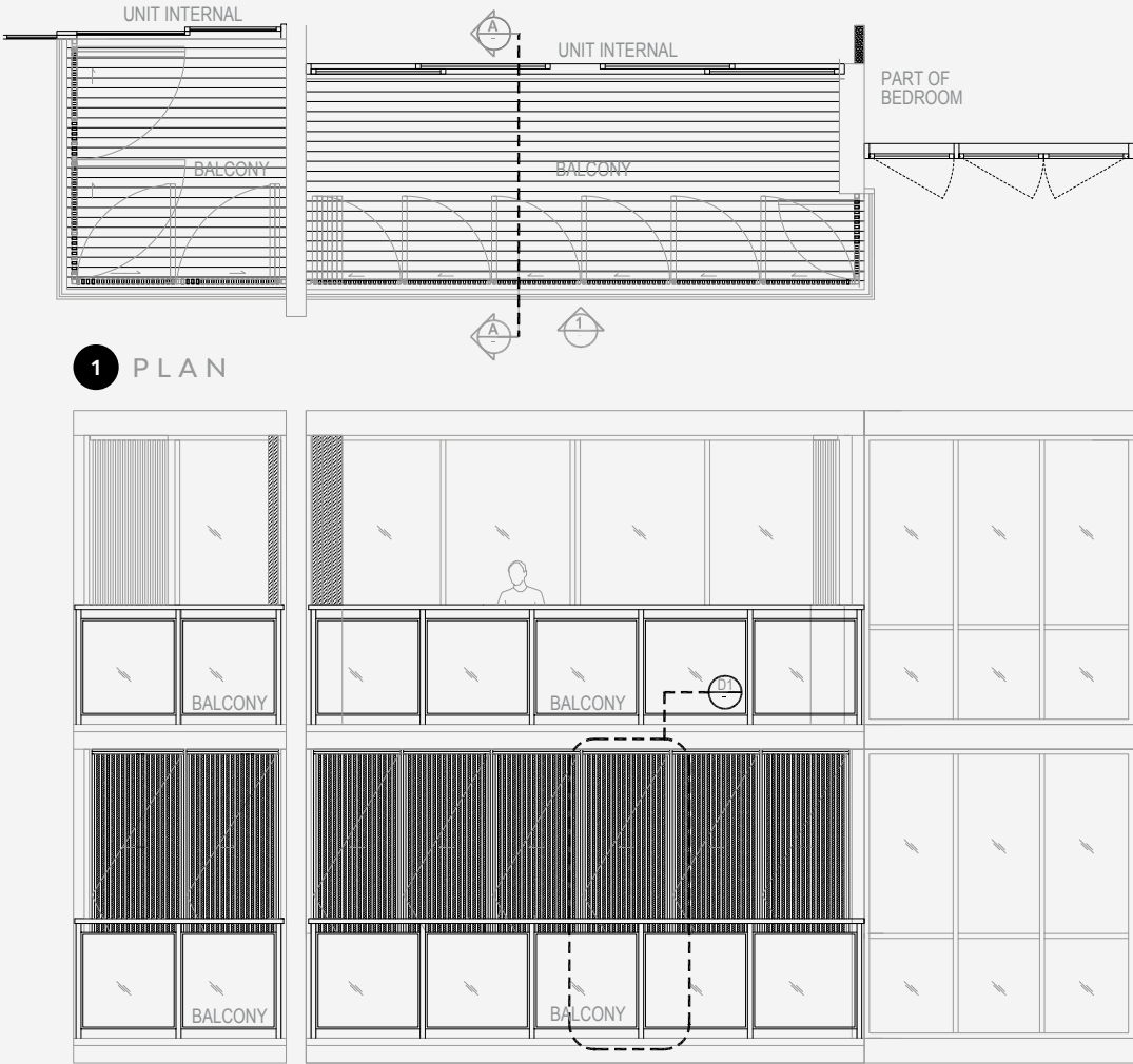
2 ELEVATION 1
